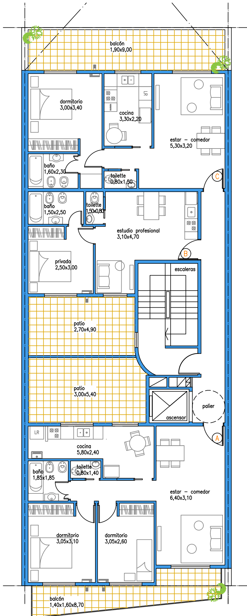
MEDRANO 458 - PLANTA 1º PISO
