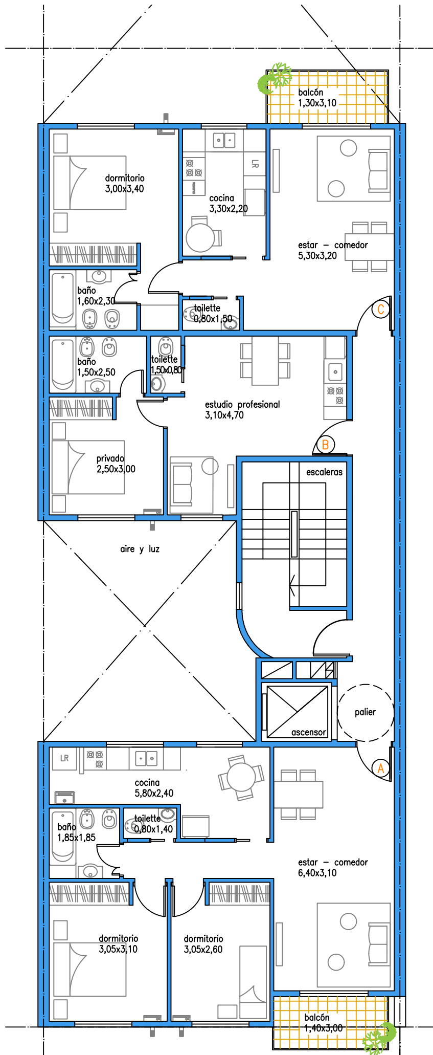
MEDRANO 458 - PLANTA TIPO 2º A 6º PISO
