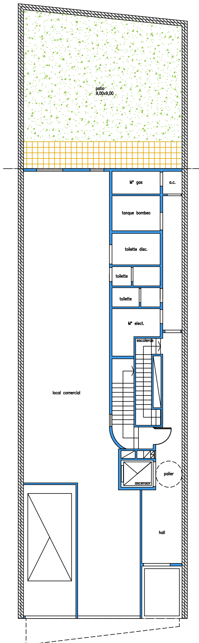
MEDRANO 458 - PLANTA BAJA
