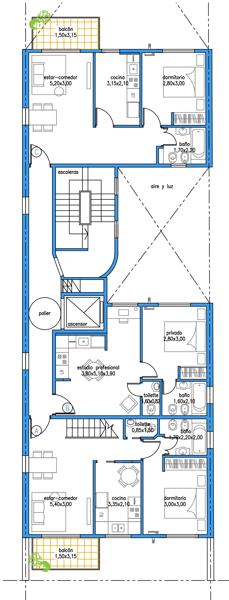
ACUÑA DE FIGUEROA 455 - PLANTA 7º PISO
