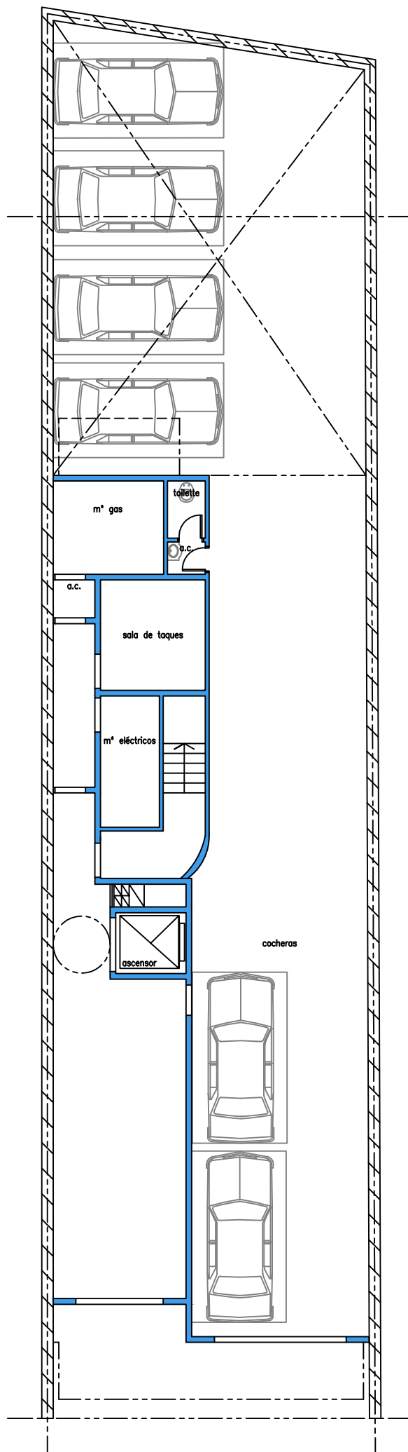
ACUÑA DE FIGUEROA 455 - PLANTA BAJA
