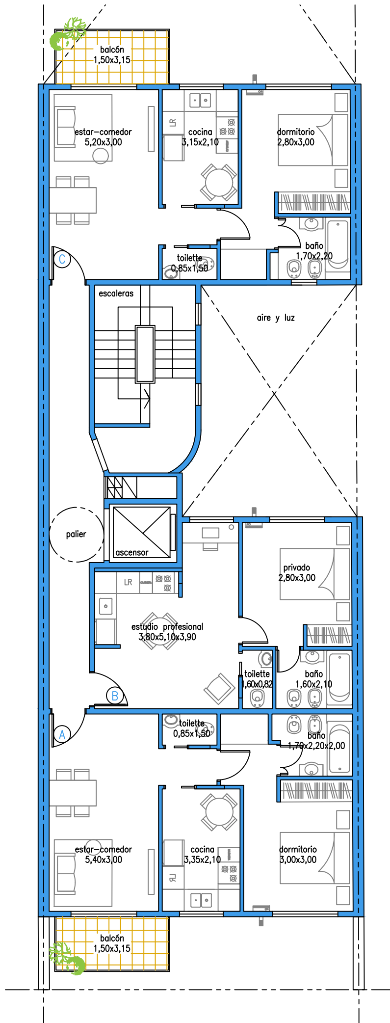
ACUÑA DE FIGUEROA 455 - PLANTA TIPO 2º A 6º PISO
